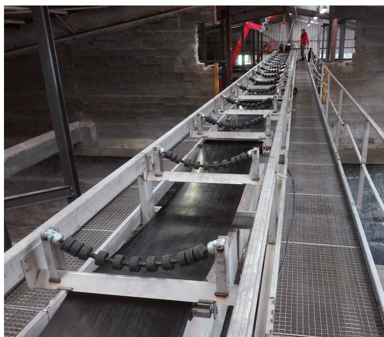
Transporteur à bande pour engrais Construction inox et limberoller
